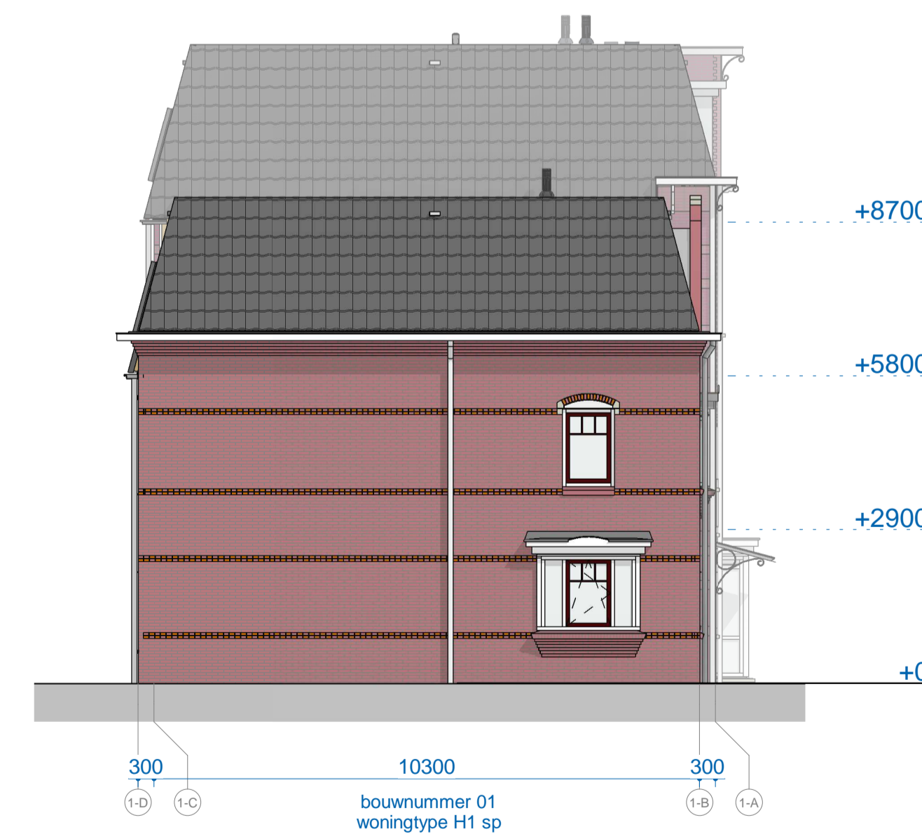
B1 linkergevel
