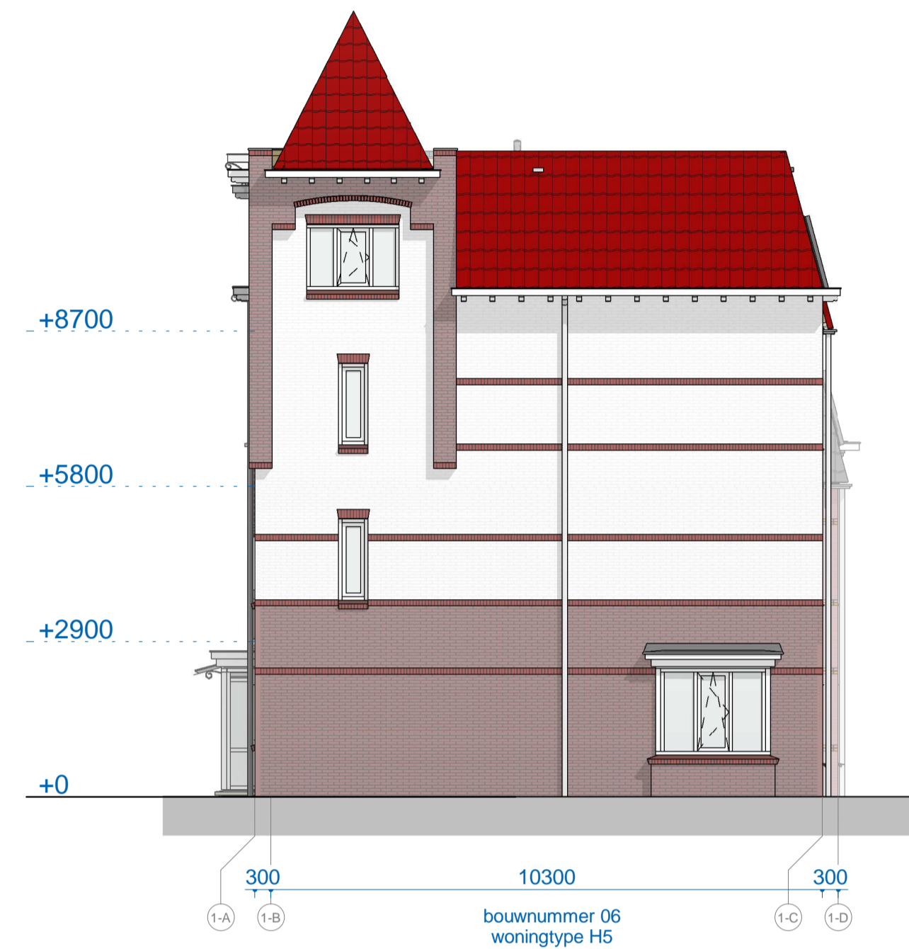
B1 rechtergevel
