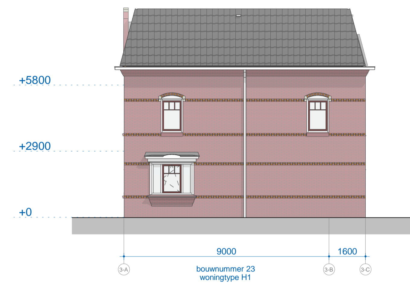
B5 rechtergevel 1:100
