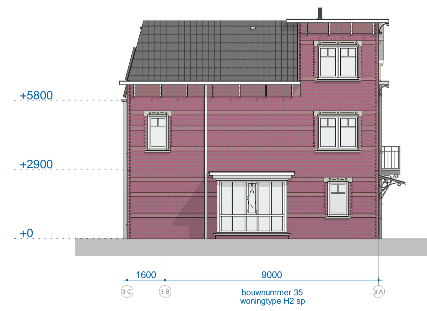
B5 linkergevel 1:100
