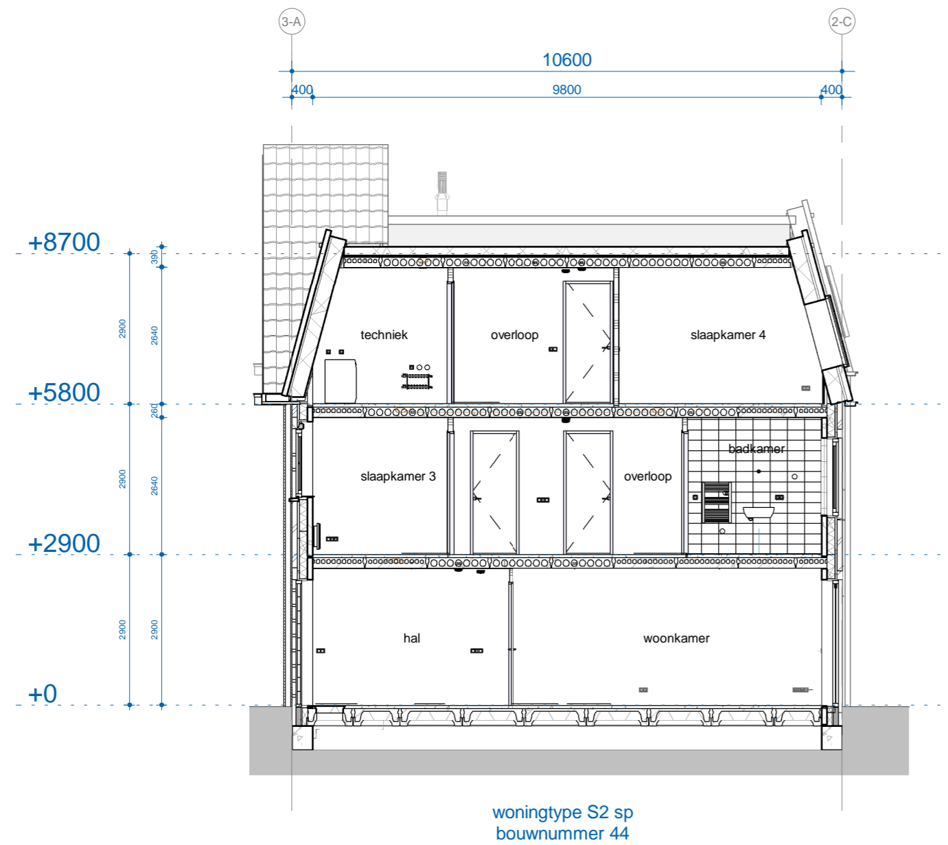
B7 doorsnede A
