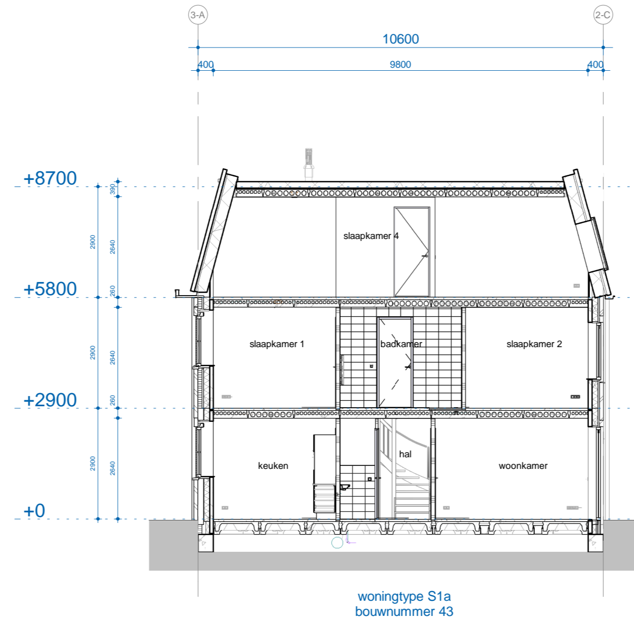
B7 doorsnede B
