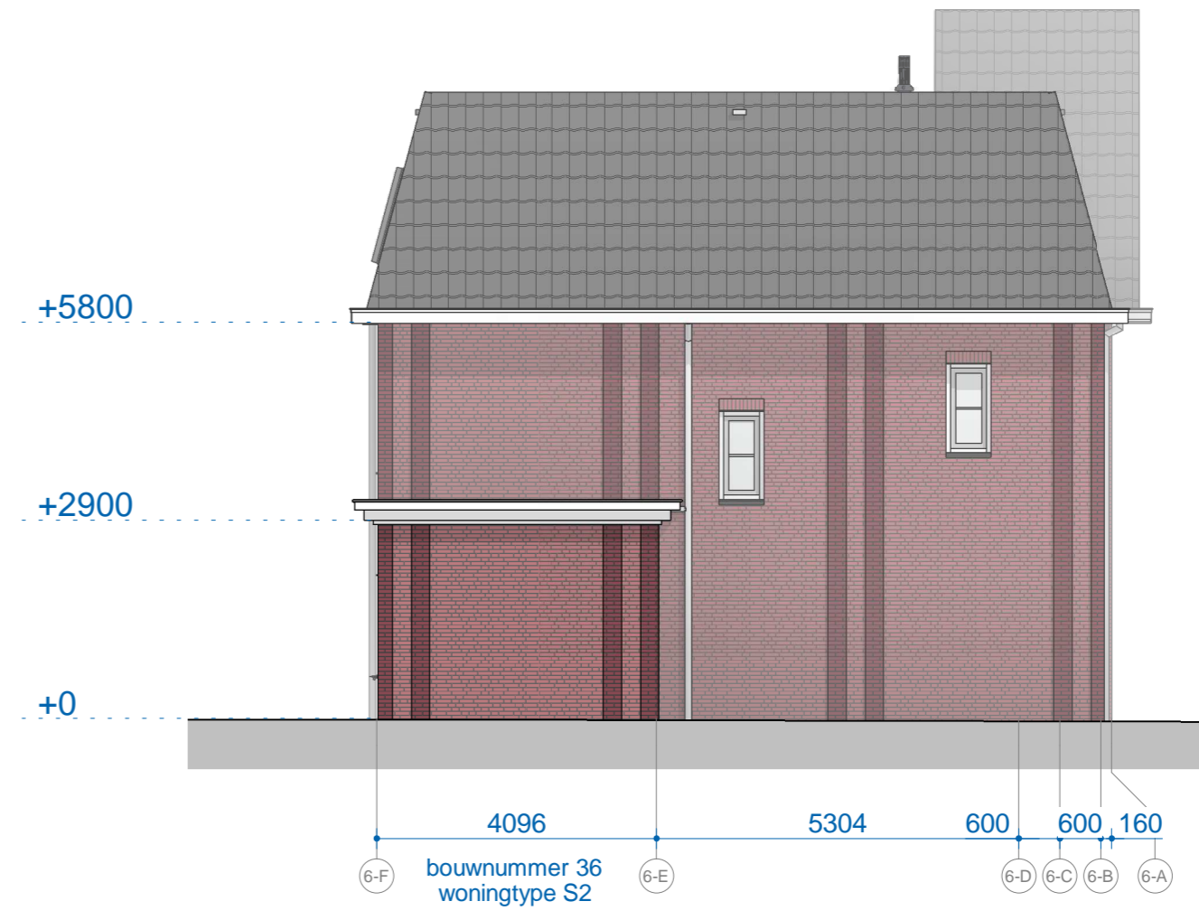
B6 linkergevel 1 : 100
