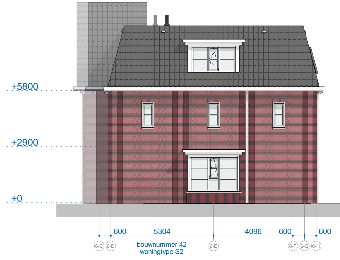
B6 rechtergevel 1 : 100
